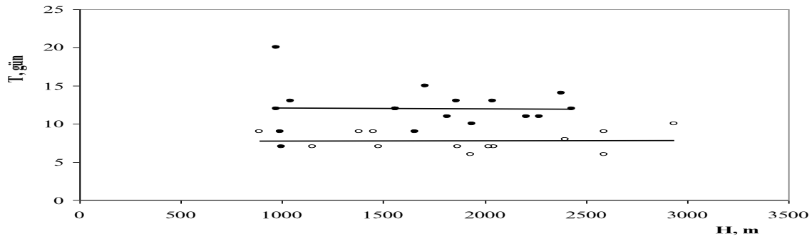
Şəkil 1. Daşqının davamiyyəti ilə hündürlük arasında əlaqə qrafiki.
