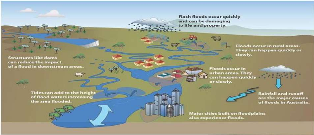
Şəkil 2. Daşqın hadisəsinə meteoroloji amillərin təsiri
