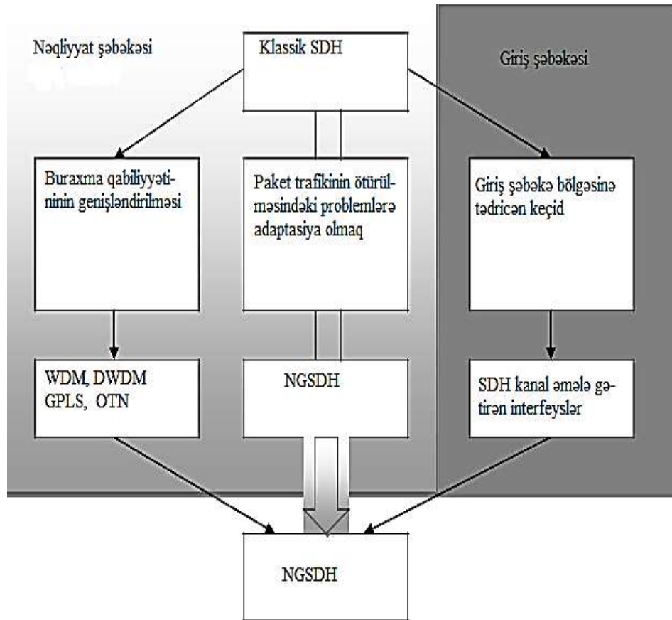
Şəkil 7. NGSDH texnologiyasının inkişafının əsas istiqamətləri
