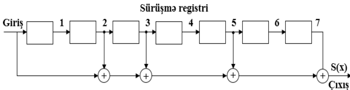
Şəkil 1. CRC hesabının realizəsi sxemi
