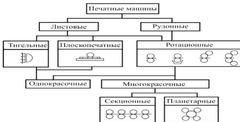
Рис. 2. Классификация печатных машин
