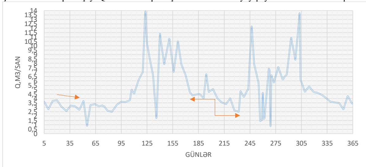
Şəkil 2. Dəmiraparaçay-Qəbələ məntəqəsi üçün 2005-ci il üzrə yay-payız azsulu dövr hidroqrafı
