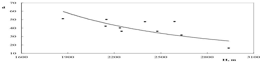
Şəkil 2. Böyük Qafqaz çaylarının daşqınlıq əmsalının hündürlükdən asılılıq qrafiği
